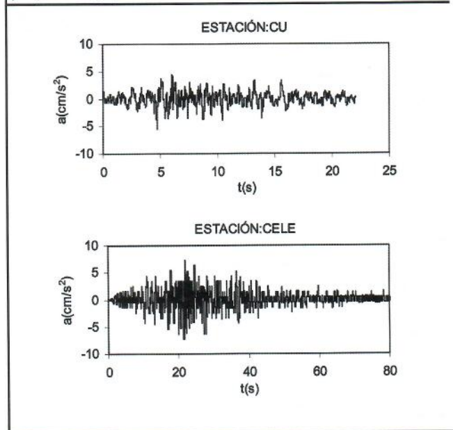
Figura 1. Acelerogramas correspondientes al temblor del 10 de diciembre de 1994 (componente NS) registrados en la estaciones CELE y CU.
