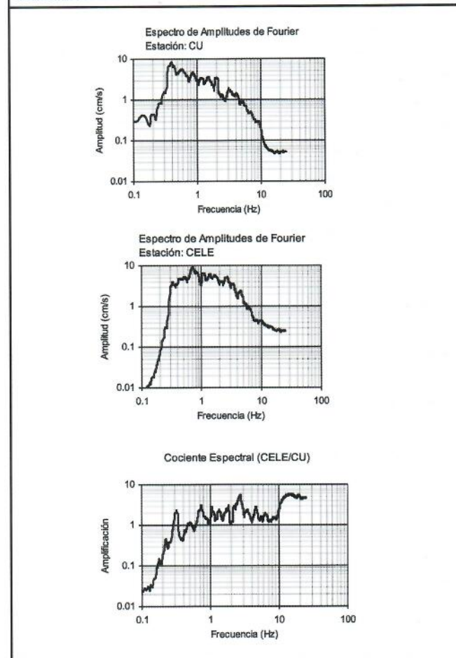
Figura 2. Espectros de Fourier y cociente espectral correspondientes al temblor del 10 de diciembre de 1994.
