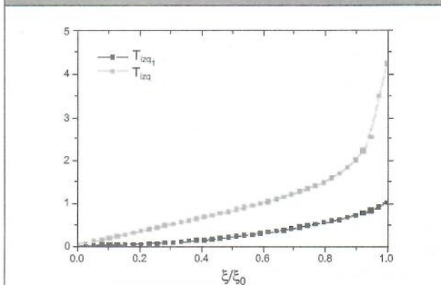
FIGURA 6. GRADIENTES DE TEMPERATURA EN LA PARED IZQUIERDA, CORRESPONDIENTE AL CASO DE LA FIGURA 5. LA CURVA SUPERIOR CORRESPONDE A G_s Y LA CURVA INFERIOR A G_f .
