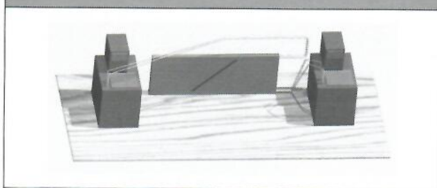
FIGURA 8. ARREGLO EXPERIMENTAL DE PLACA DE COBRE CON UNA FRACTURA INCLINADA LLENA DE FLUIDO.
