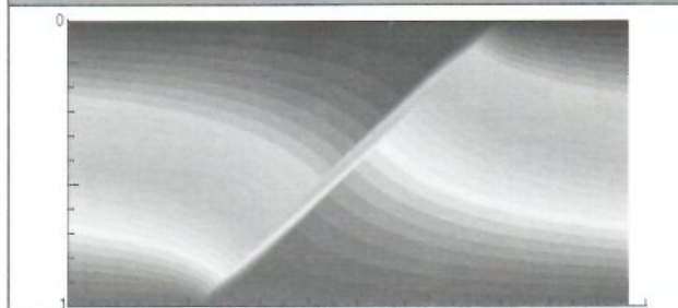
FIGURA 5. DISTRIBUCIÓN DE TEMPERATURAS EN Y ALREDEDOR DE UNA FRACTURA INCLINADA A 45 GRADOS CON k_s \gg k_f Y VISCOSIDAD ALTA.
