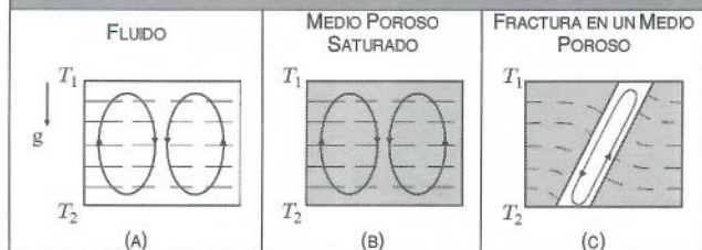
FIGURA 1. PATRONES DEL MOVIMIENTO CONVECTIVO (CURVAS CERRADAS). EN A) UNA CAPA FLUIDA B) UN MEDIO POROSO SATURADO Y C) UNA FRACTURA INCLINADA. EN LOS CASOS A) Y B) EL MOVIMIENTO INICIA EN VALORES BIEN DEFINIDOS (CRÍTICOS) DEL NÚMERO DE RAYLEIGH MIENTRAS QUE EN C) EL MOVIMIENTO OCURRE PARA CUALQUIER VALOR DE ESTE NÚMERO.
