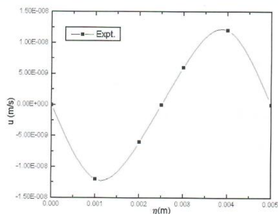
FIGURA 10. GRÁFICA DEL PERFIL DE VELOCIDADES (CURVA CONTINUA) DADA POR LA ECUACIÓN (29). LOS PUNTOS EXPERIMENTALES FUERON OBTENIDOS MEDIANTE MEDICIONES DE VIP.
