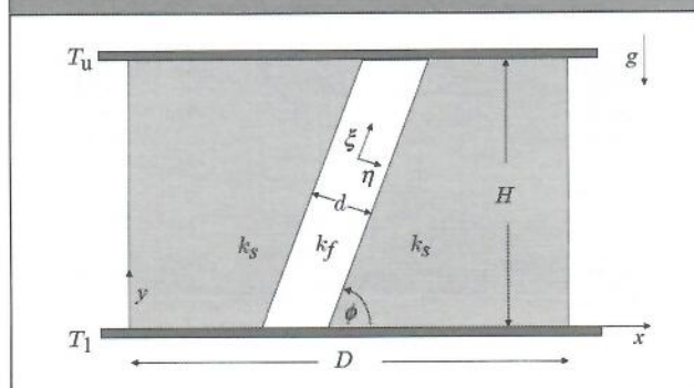
FIGURA 3. REPRESENTACIÓN GRÁFICA DE UNA FRACTURA INCLINADA. EL GRADIENTE VERTICAL EN LOS EXTREMOS VERTICALES, COMO EN LOS YACIMIENTOS ES G=(T_1-T_u)/H .
