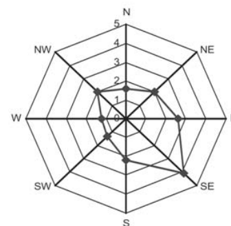
Gráfica 2. Dirección y velocidad del viento (M/S) en Toluca.
