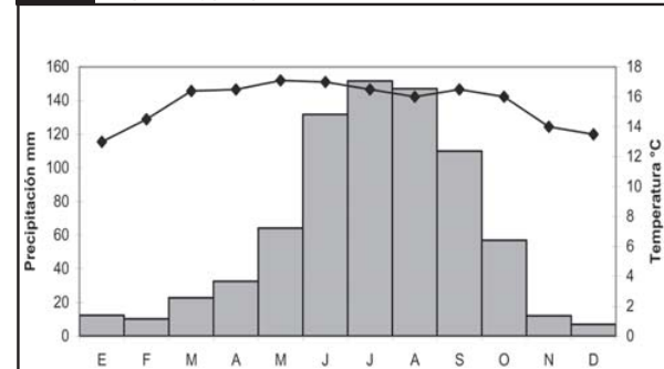
Gráfica 3. Temperatura y precipitación media mensual en Toluca centro.
