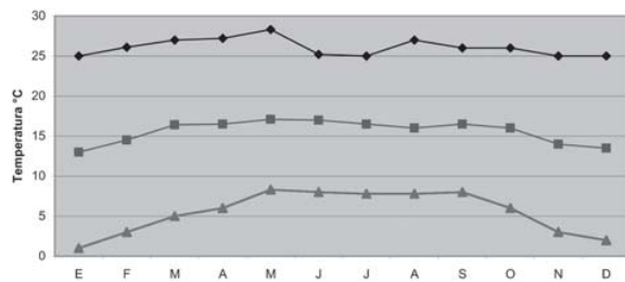
Gráfica 1. Temperaturas máximas, media y mínimas en el centro de Toluca.
